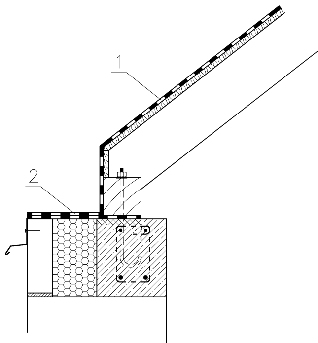
Obr. 4 - Napojenie parozábrany na obvodové murivo – odkvapová hrana 1 - Parozábrana z asfaltovaného pásu, 2 - nalepenie alebo natavenie na pripravený prírez z asfaltovaného pásu
