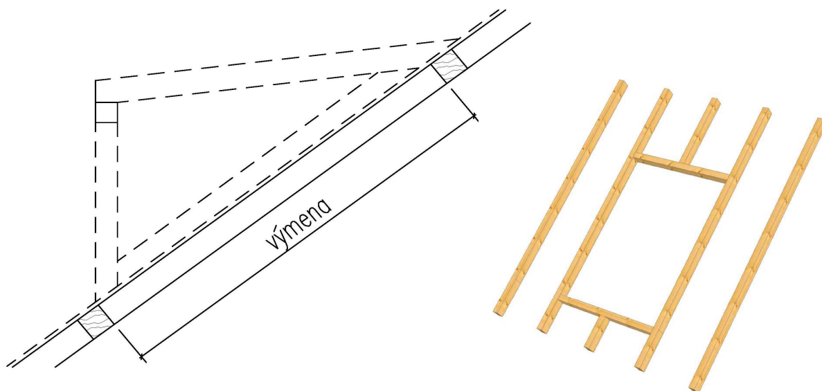
Obr. 20 - Umiestnenie výmeny krovu pri pultovom vikieri
