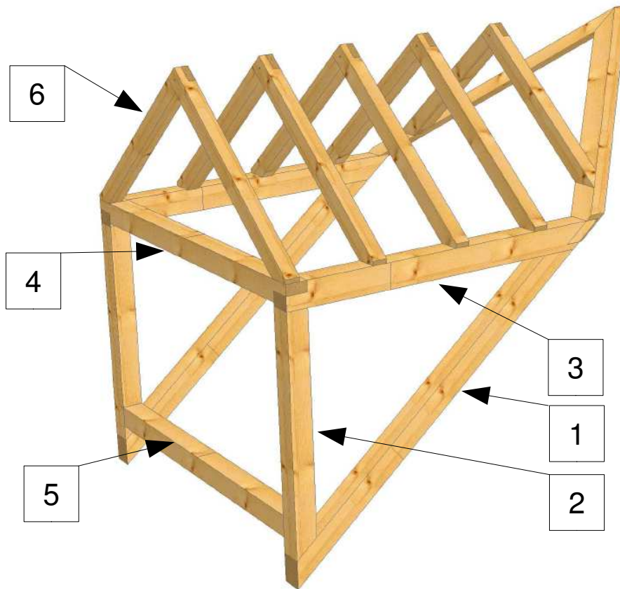
Obr. 24 - Konštrukcia sedlového vikiera (1 - základný bočný diel, 2 - stĺp, 3 - pomúrnicca, 4 - nadpražný diel, 5 - parapetný diel, 6 - krokvy)
